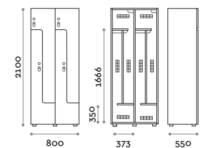
VANB48-23 Doppia colonna 4 ante a "L" Double column locker, 4 L-shaped doors
